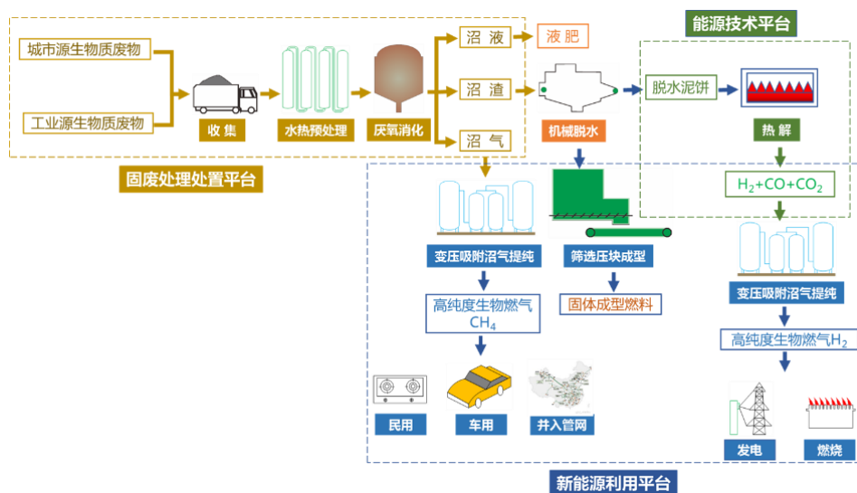
图 1 生物质废物清洁燃气工艺流程图
