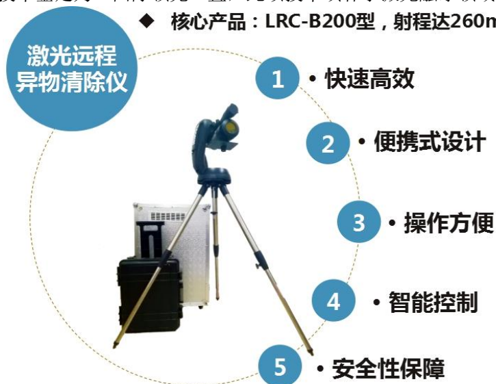
图 1 便携式激光除电网异物装置
